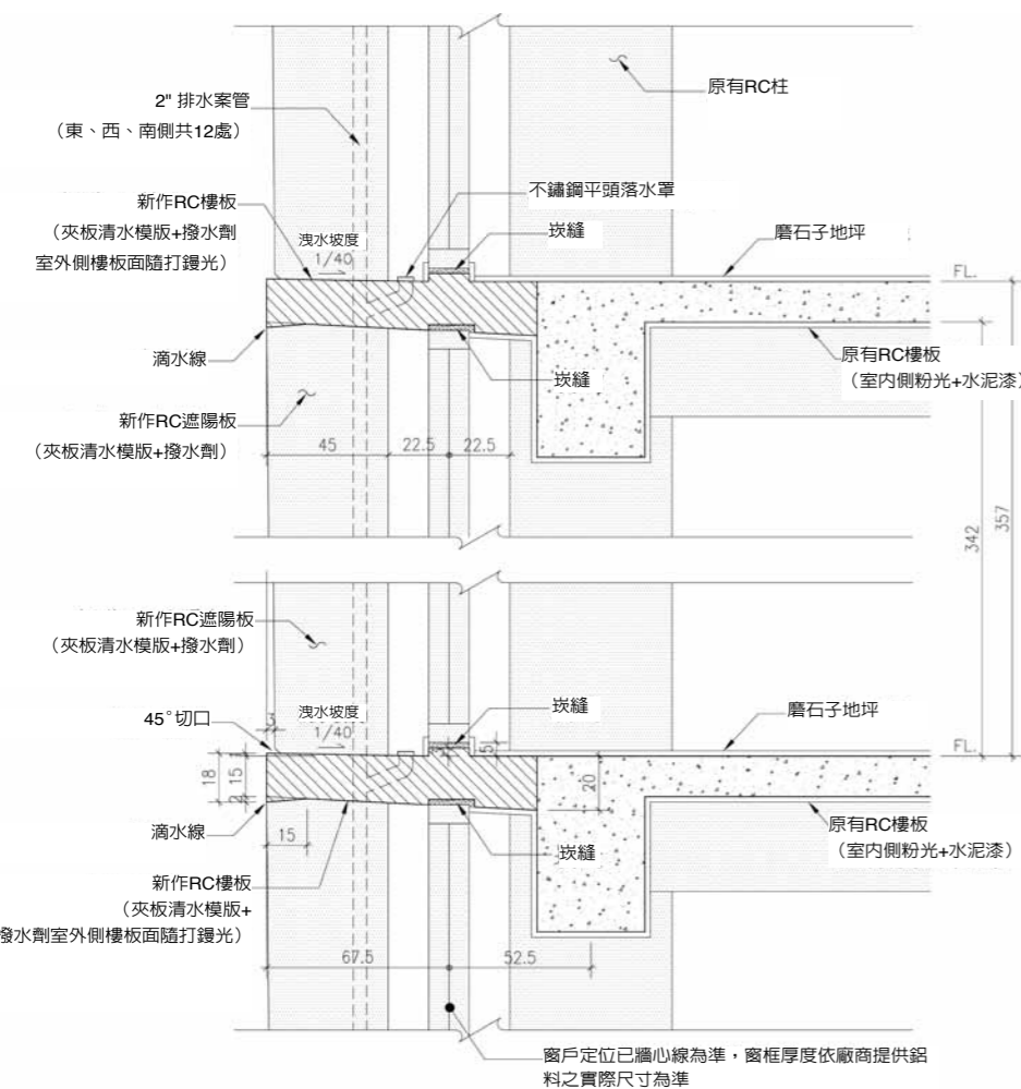
B棟雨遮樓版剖面標準圖 Scale = 1/60
